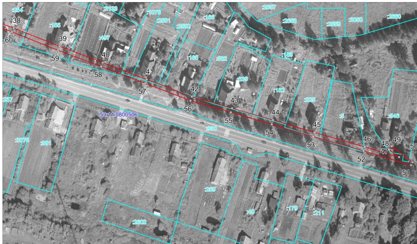
ВЛ-0,4 кВ Л-1 от КТП Ермолино-5
